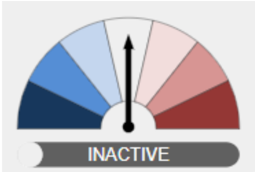
ENSO Outlook
